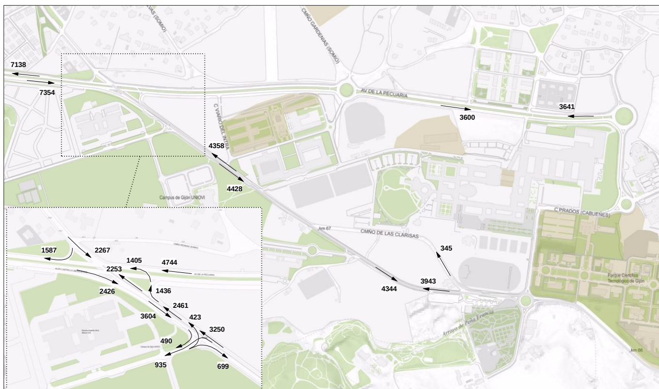
Figura 25. Datos de estaciones de aforo. Año 2019. IMD
