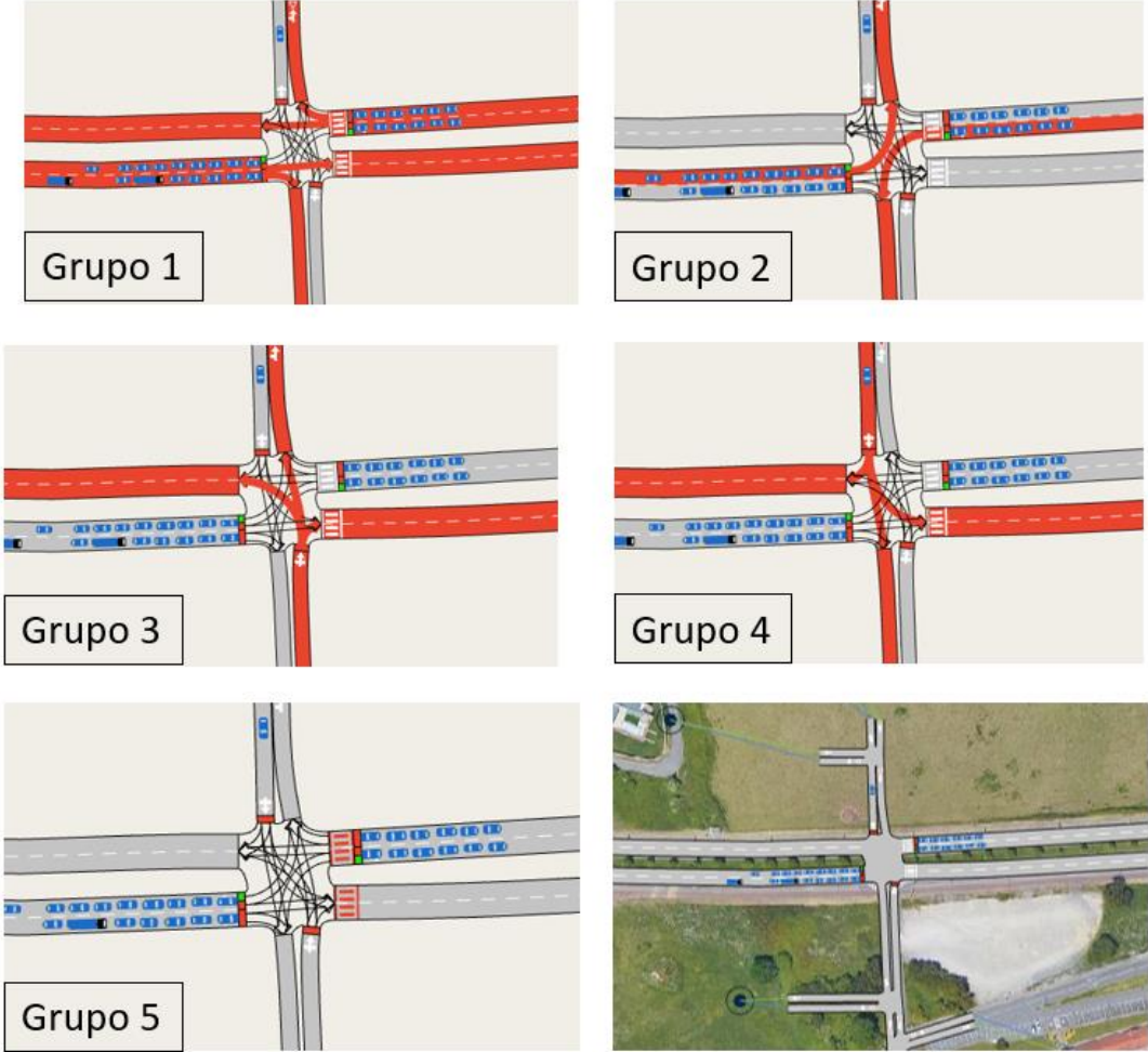
Figura 47. Futura intersección semaforizada, acceso a los nuevos desarrollos en avenida de la Pecuaria
