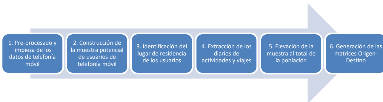
Figura 13. Pasos para el tratamiento de los datos móviles
