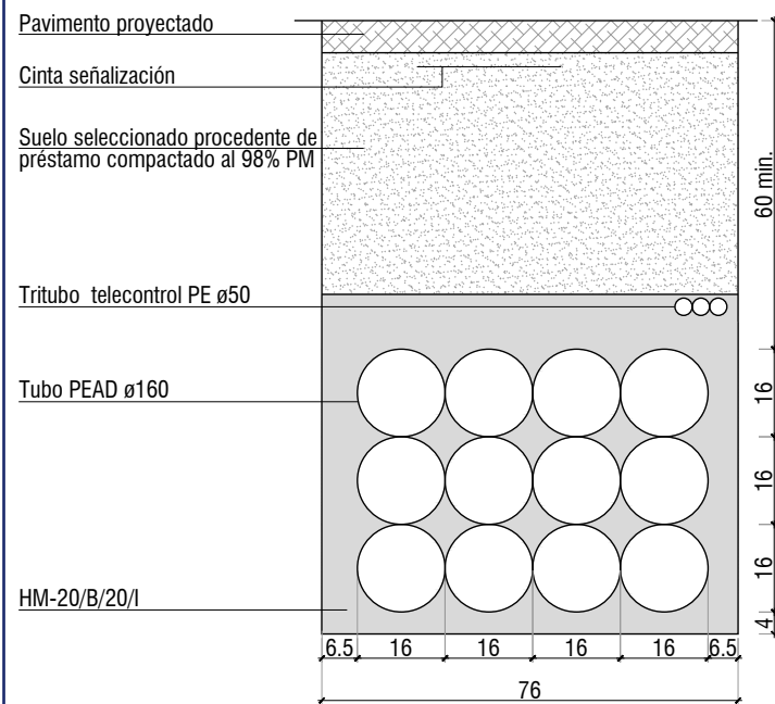
ZANJA DE 12 TUBOS BAJO ACERA 1/15 (cotas en cm)
