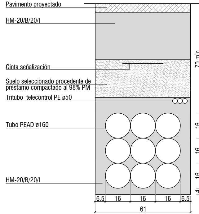
ZANJA DE 9 TUBOS BAJO APARCAMIENTO 1/15 (cotas en cm)
