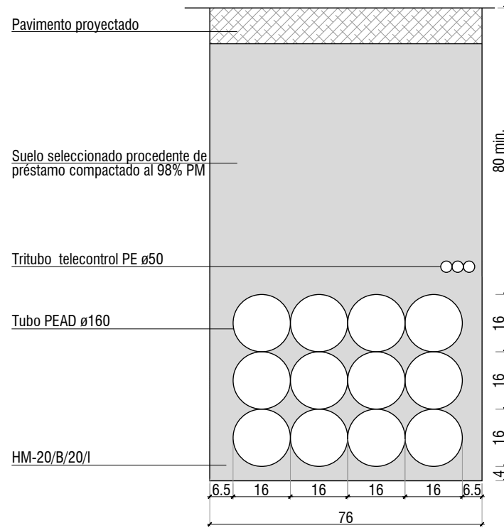
ZANJA DE 12 TUBOS BAJO CALZADA 1/15 (cotas en cm)
