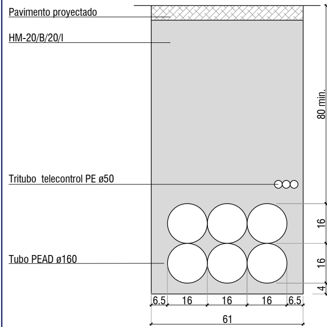
ZANJA DE 6 TUBOS BAJO CALZADA 1/15 (cotas en cm)
