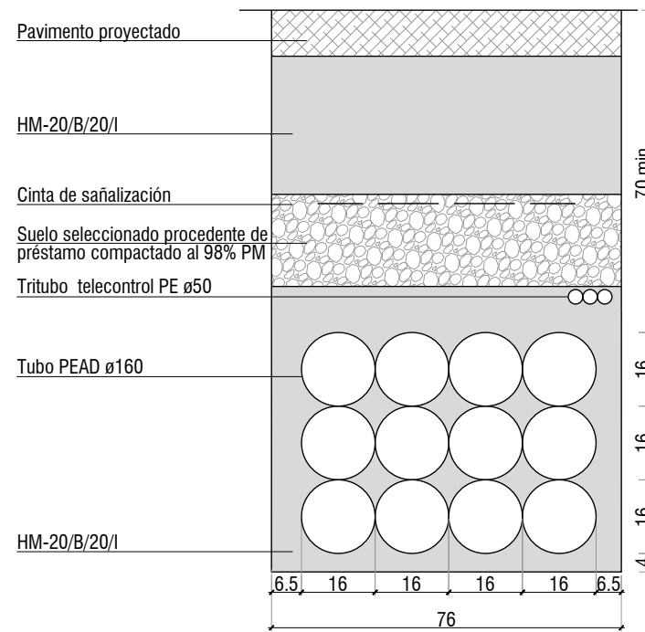
ZANJA DE 12 TUBOS BAJO APARCAMIENTO 1/15 (cotas en cm)
