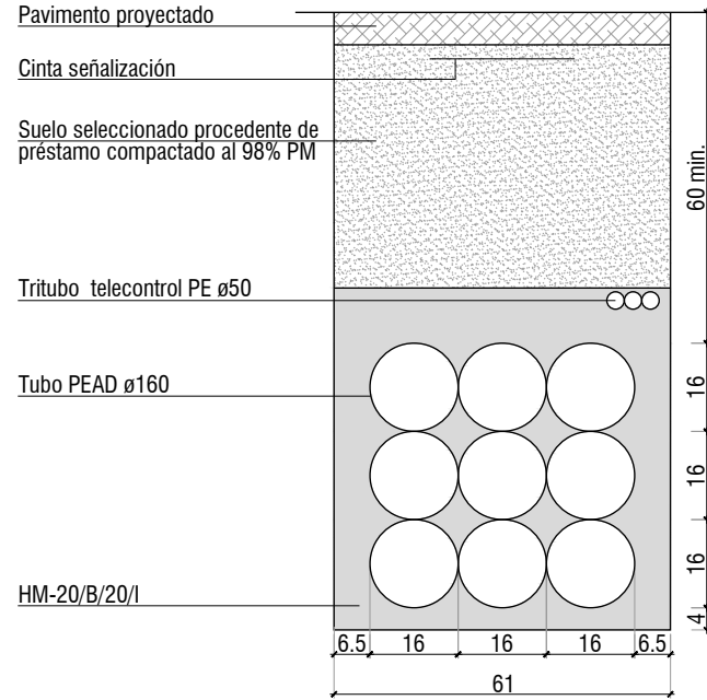
ZANJA DE 9 TUBOS BAJO ACERA 1/15 (cotas en cm)
